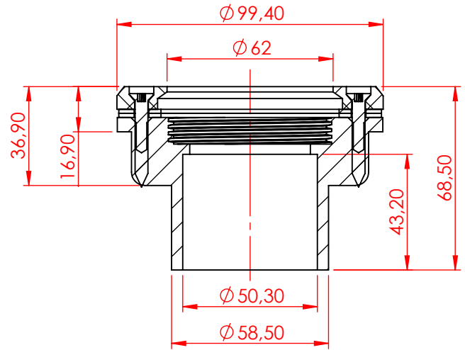
SEÇÃO A-A
